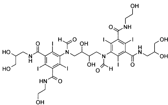
Formula (IIIk)
