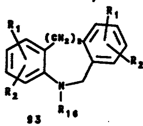
93 (R 16 -H) 5,6,11,12-tetrahydridibenz[b,f]azecine
