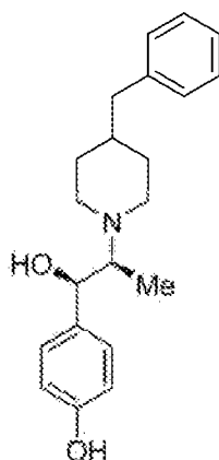
ifenprodil
