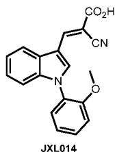
(E)-2-Cyano-3-(1-(2-methoxyphenyl)-1H-indol-3-yl)acrylic acid (JXL014)
