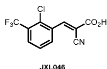
( E )-3-(2-chloro-3-(trifluoromethyl)phenyl)-2-cyanoacrylic acid (JXL046)
