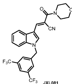
( E )-3-(1-(3,5-Bis(trifluoromethyl)benzyl)-1 H -indol-3-yl)-2-(morpholine-4-carbonyl)acrylonitrile (JXL081)
