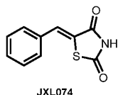
(Z)-5-Benzylidenethiazolidine-2,4-dione (JXL074)
