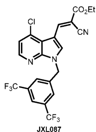
Ethyl ( E )-3-(1-(3,5-bis(trifluoromethyl)benzyl)-4-chloro-1 H -pyrrolo[2,3- b ]pyridin-3-yl)-2-cyanoacrylate (JXL087)
