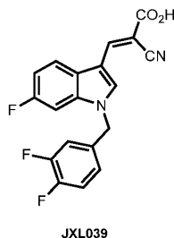
(E)-2-Cyano-3-(1-(3,4-difluorobenzyl)-6-fluoro-1H-indol-3-yl)acrylic acid (JXL039)
