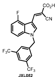
( E )-3-(1-(3,5-Bis(trifluoromethyl)benzyl)-4-fluoro-1 H -indol-3-yl)-2-cyanoacrylic acid (JXL052)
