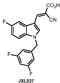
(E)-2-Cyano-3-(1-(3,5-difluorobenzyl)-5-fluoro-1H-indol-3-yl)acrylic acid (JXL037)
