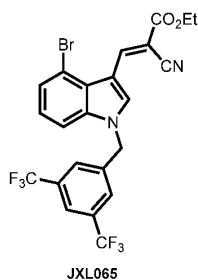
Ethyl (E)-3-(1-(3,5-bis(trifluoromethyl)benzyl)-4-bromo-1H-indol-3-yl)-2-cyanoacrylate (JXL065)
