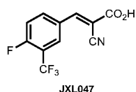
( E )-2-cyano-3-(4-fluoro-3-(trifluoromethyl)phenyl)acrylic acid (JXL047)
