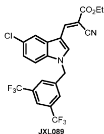
Ethyl ( E )-3-(1-(3,5-bis(trifluoromethyl)benzyl)-5-chloro-1 H -indol-3-yl)-2-cyanoacrylate (JXL089)
