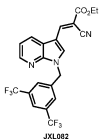
Ethyl ( E )-3-(1-(3,5-bis(trifluoromethyl)benzyl)-1 H -pyrrolo[2,3-b]pyridin-3-yl)-2-cyanoacrylate (JXL082)
