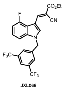
Ethyl ( E )-3-(1-(3,5-bis(trifluoromethyl)benzyl)-4-fluoro-1 H -indol-3-yl)-2-cyanoacrylate (JXL066)
