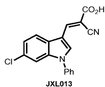
(E)-3-(6-Chloro-1-phenyl-1H-indol-3-yl)-2-cyanoacrylic acid (JXL013)
