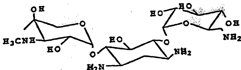
Gentamicin-B
