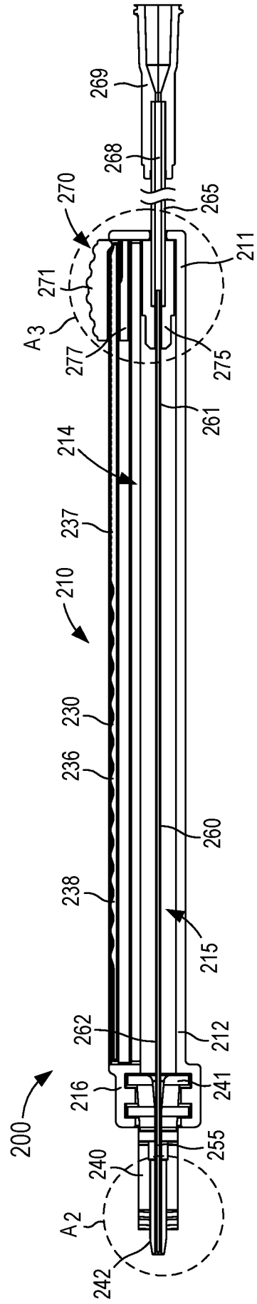
FIG. 22
