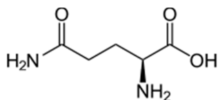
L-glutamine
