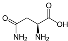
L-asparagine
