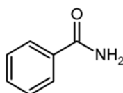
Benzamide
