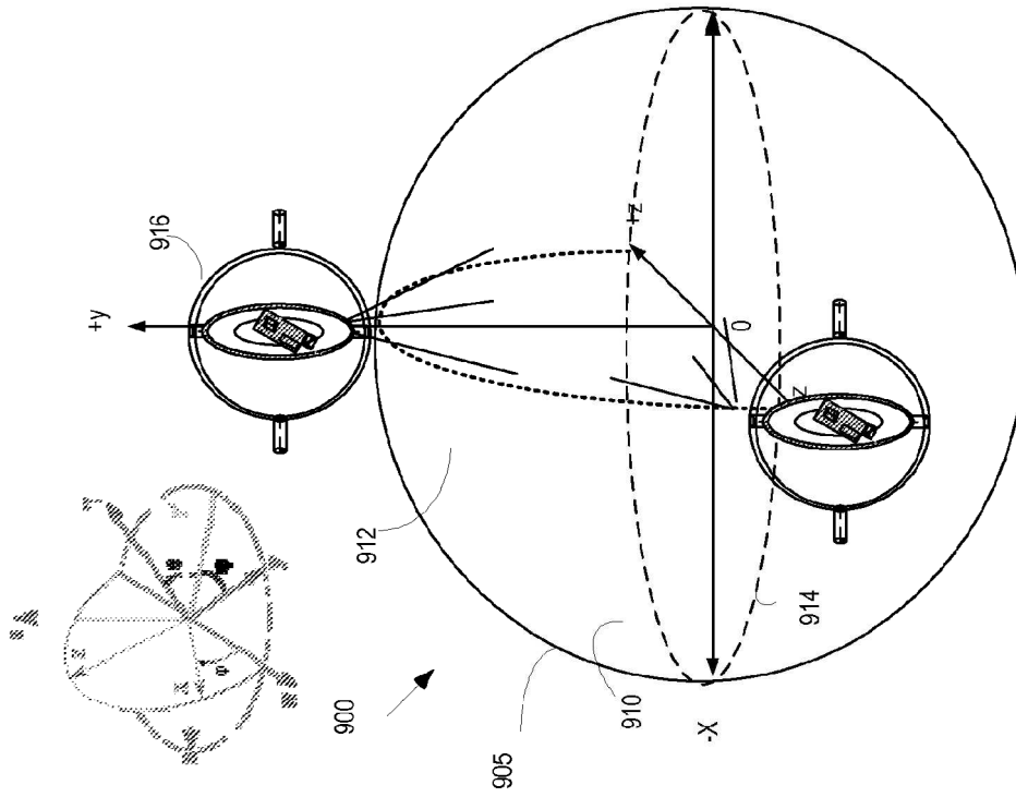
FIG. 10 PARAMETER MODELER
