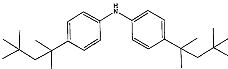
bis(4-(2,4,4-trimethylpentan-2-yl)phenyl)amine
