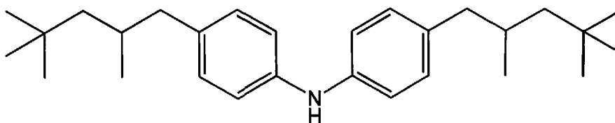
bis(4-(2,4,4-trimethylpentyl)phenyl)amine
