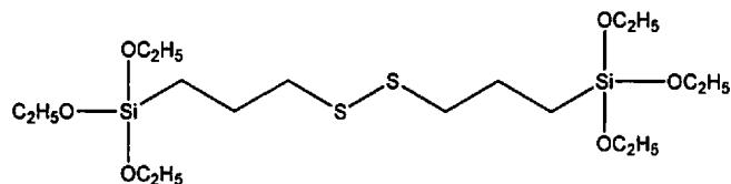
4,4,13,13-tetraethoxy-3,14-dioxa-8,9-dithia-4,13-disilahexadecane
