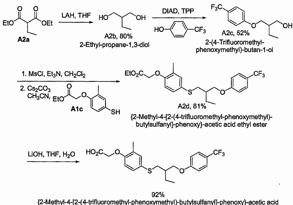
Scheme A2
