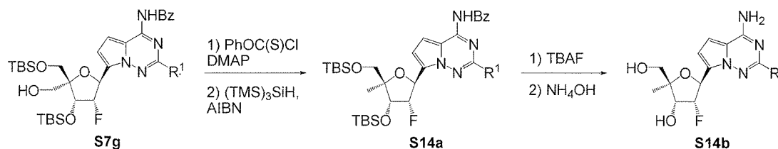
10 Scheme 14.
