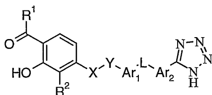
tautomer I
