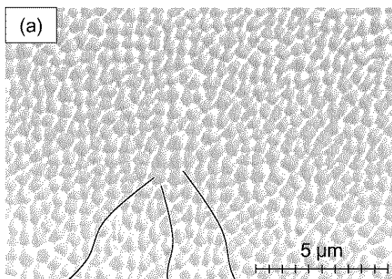
偏析セル 偏析セルの境界領域 析出強化相粒子
