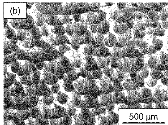
合金粉末床厚さ h = 50 \mu\text{m} レーザー光出力 P = 190 \text{ W}
