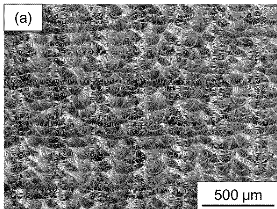
合金粉末床厚さ h = 30 \mu\text{m} レーザー光出力 P = 120 \text{ W}
