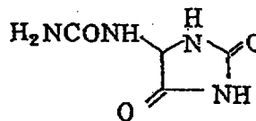
Allantoin
