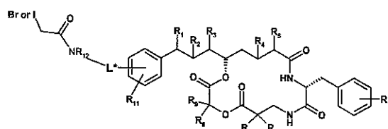
(IIa)
