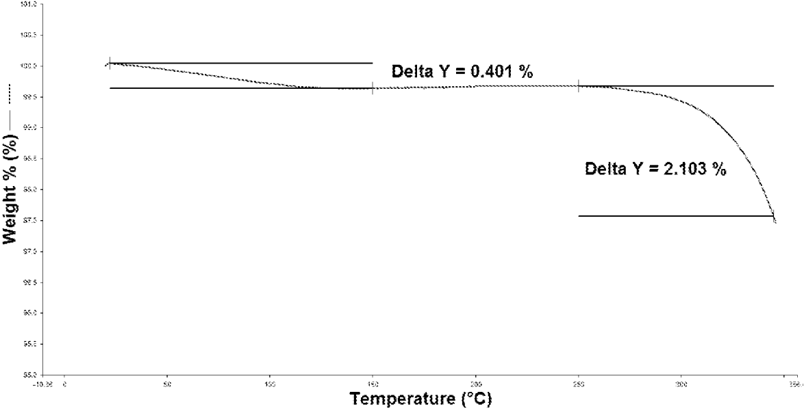
FIG. 3 TGA
