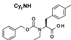
(Z-EtPhe(4-Me) Cy 2 NH)
