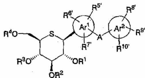
IA
