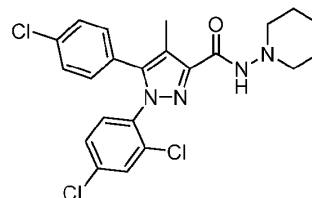
Rimonabant
