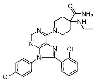
Otenabant
