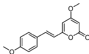
Yangonin
