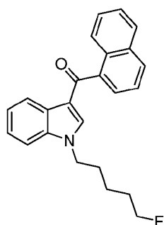
AM-2201
