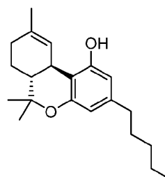
Dronabinol
