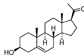
Pregnenolone
