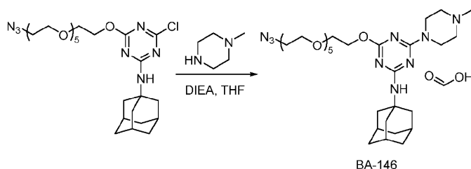
BA-146
