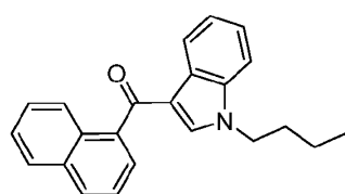
JWH-073
