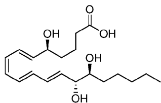
Lipoxin A4
