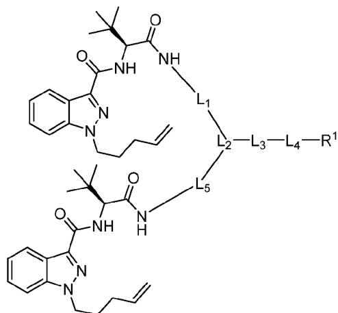
Formula (V-a)
