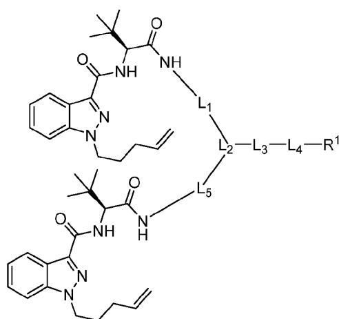
Formula (V-a)
