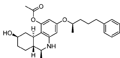
Levonantradol
