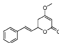
Kavain
