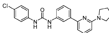
PSNCBAM-1
