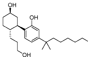
CP 55,940
