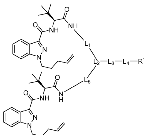
Formula (V-a)
