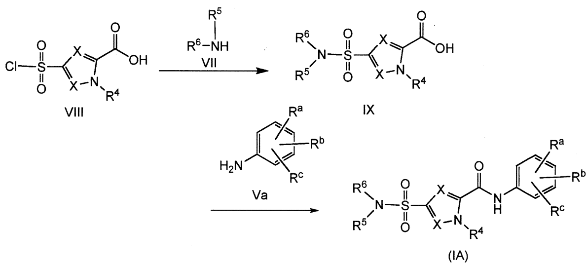
Scheme 2a
