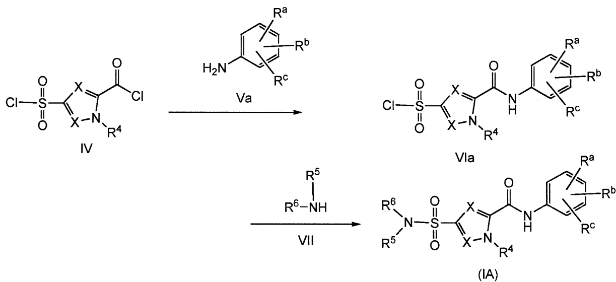
Scheme 1a
