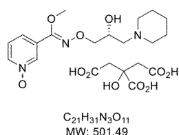
Methoxylated ORZY-04 (RRT 0.74)
