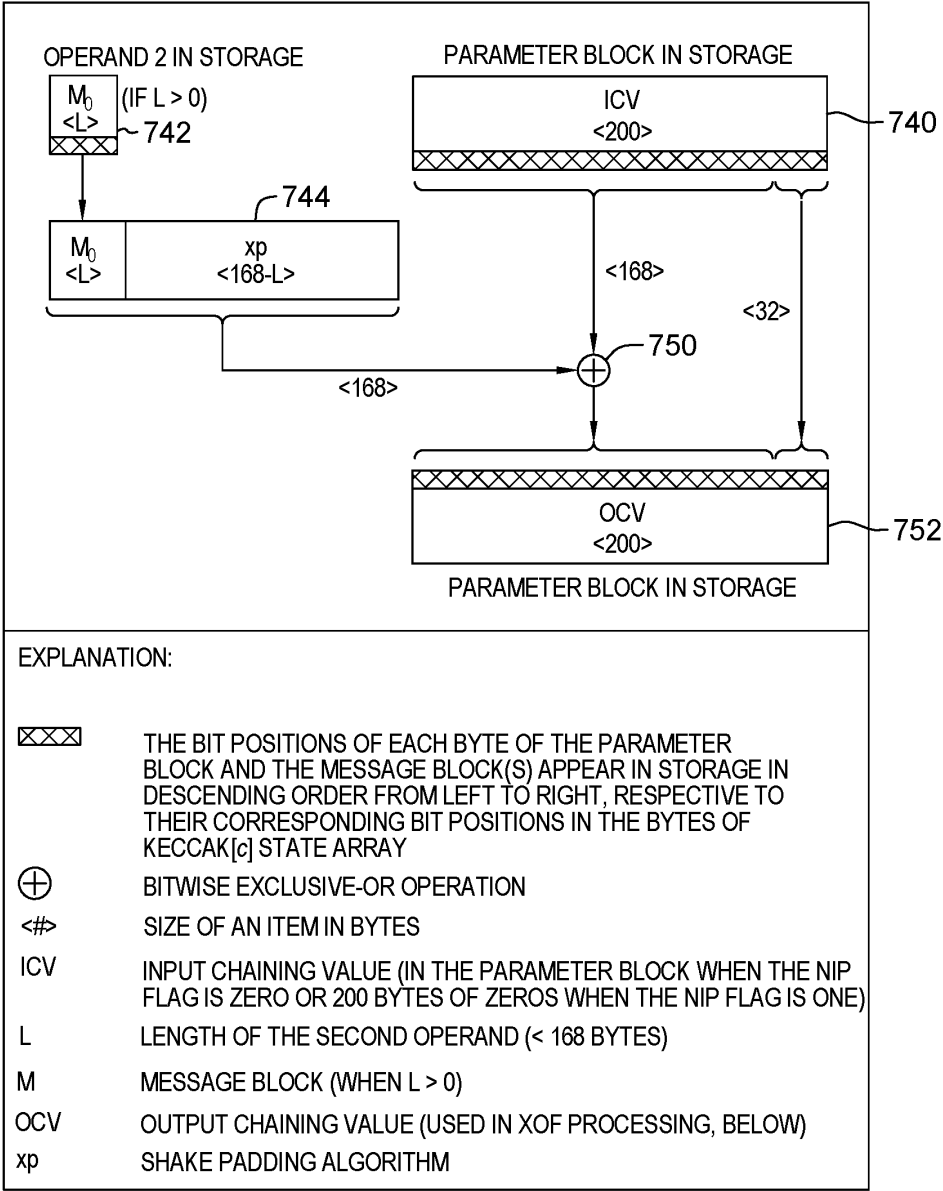
KLMD-SHAKE-128 PADDING ( L < 168 )
