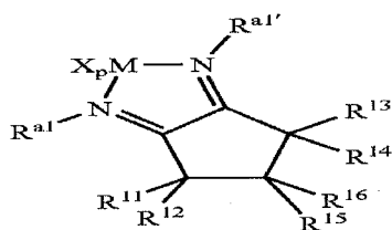
Structure 4e
