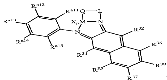
Structure 34e
