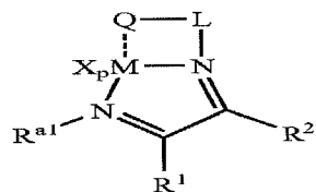
Structure 14e
