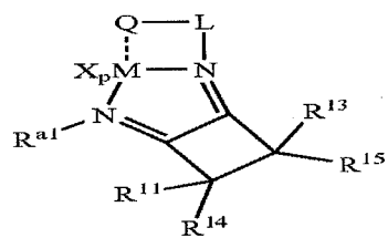
Structure 16e
