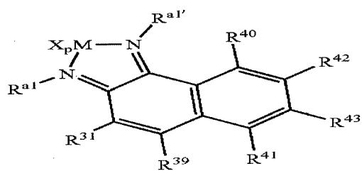
Structure 9e
