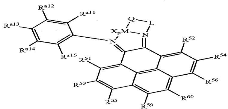
Structure 39e
