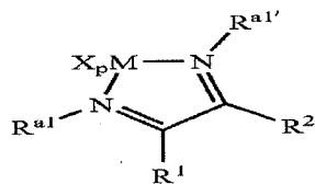
Structure 1e
