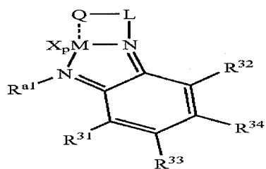
Structure 20e
