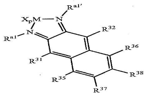
Structure 8e
