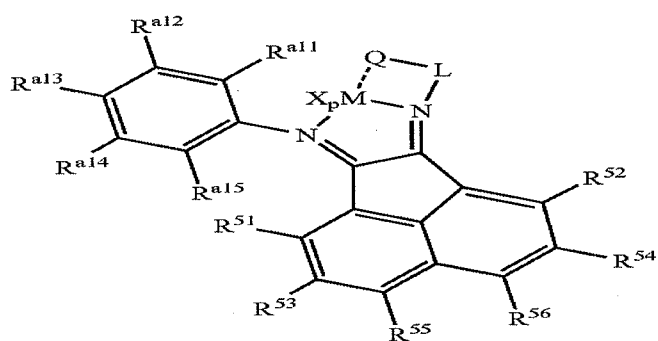
Structure 37e
