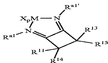
Structure 3e
