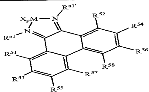
Structure 12e
