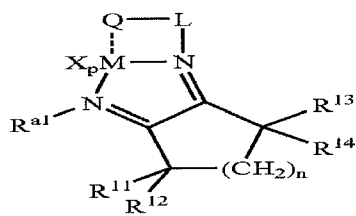
Structure 15e
