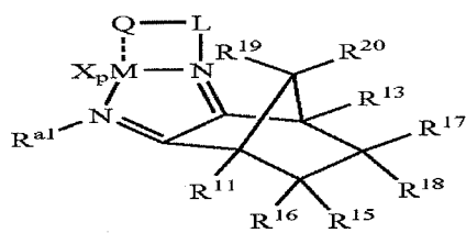
Structure 19e
