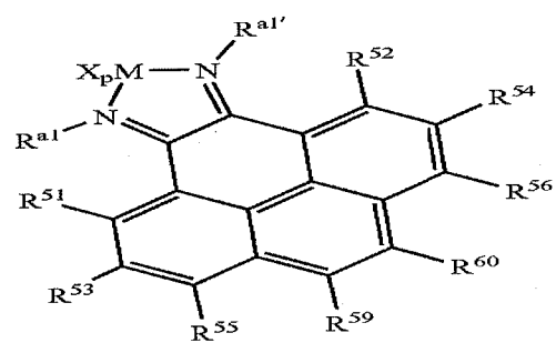
Structure 13e
