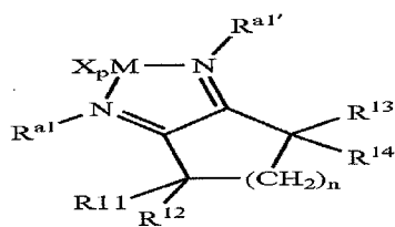
Structure 2e
