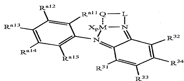
Structure 33e
