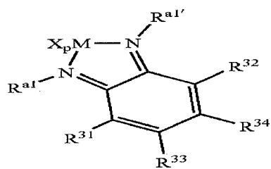
Structure 7e
