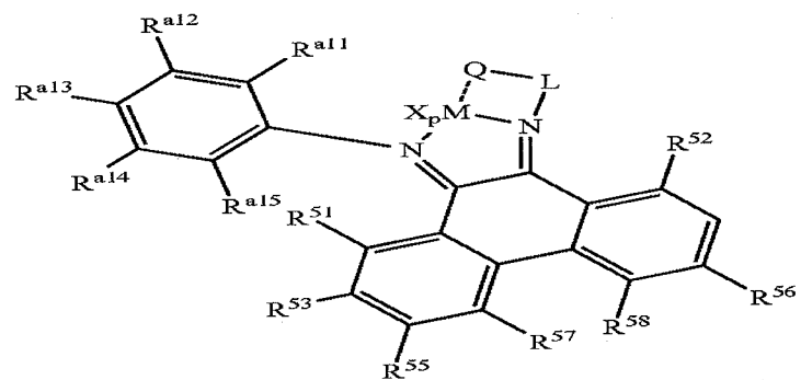
Structure 38e
