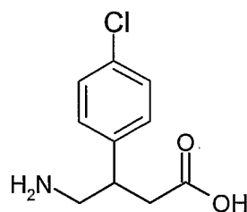
Baclofen (1)
