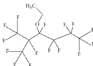
2-(Trifluoromethyl)-3-ethoxydodecafluorohexane.
