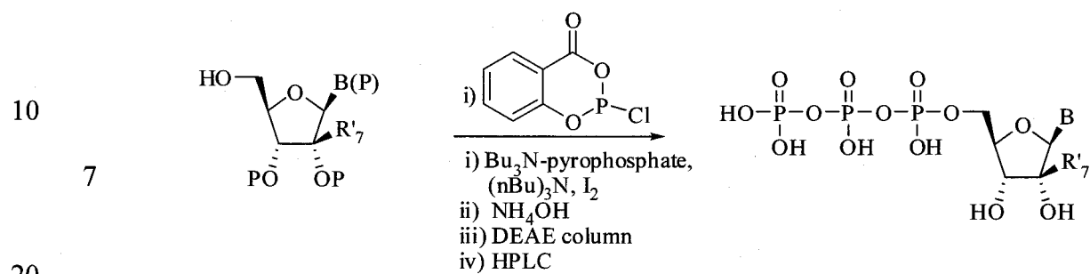
Scheme C-2.
