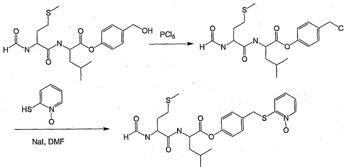
SCHEME-3
