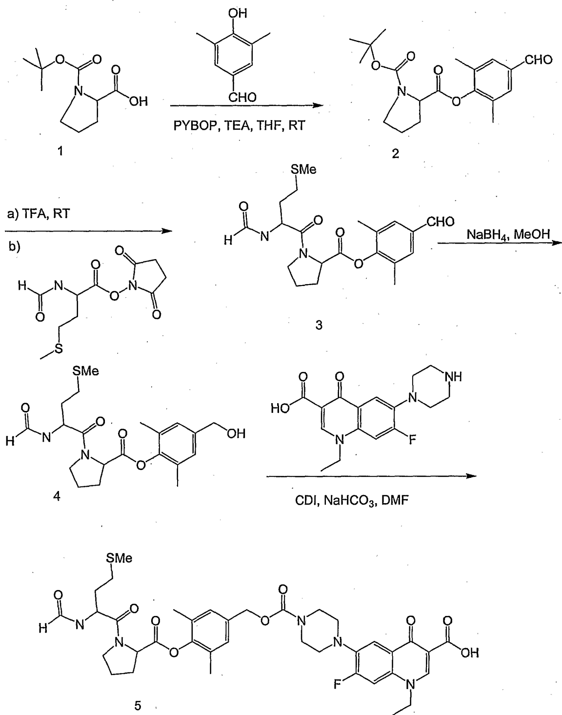
SCHEME-2
