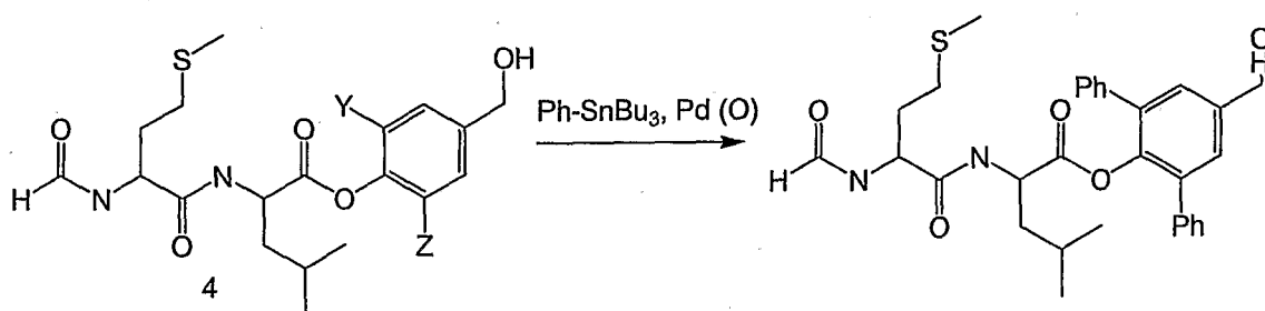
SCHEME-4
