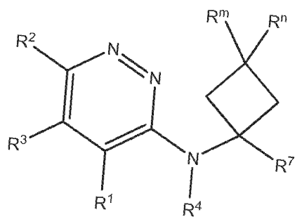
Formula XII(d)
