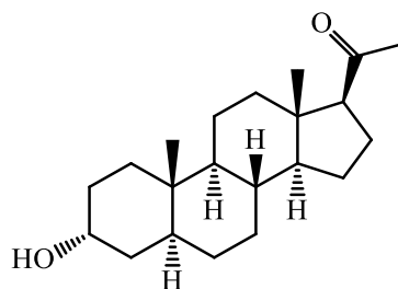
3 \alpha ,5 \alpha -Tetrahydroprogesterone Allopregnanolone
