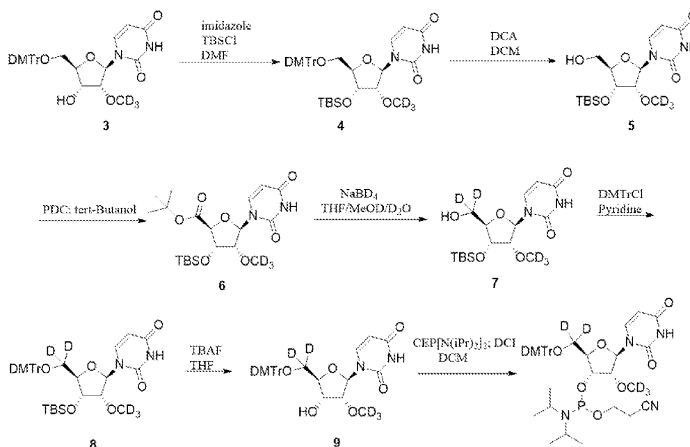
Scheme-5
