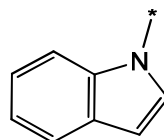
indol-1-yl
