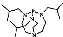
VerK B
