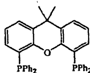
XANTPHOS
