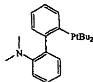
'B_A_B
