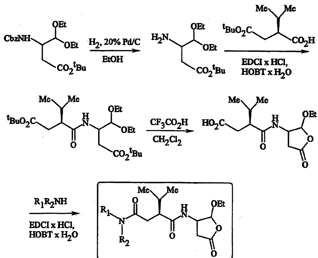
Scheme VI
