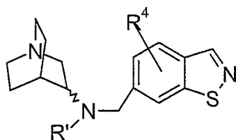
(IIIIn)
