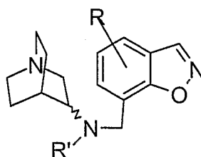
(IIIIt)
