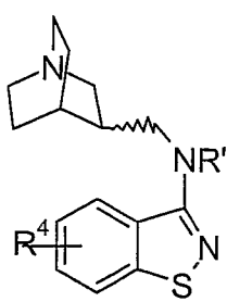
(IVj)
