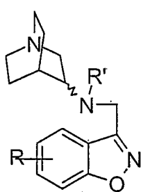
(IIIp)
