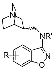
(IVp)
