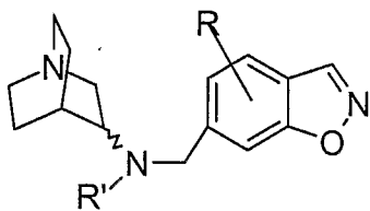
(IIIIs)
