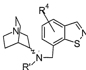
(IIIlo)
