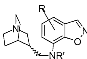
(IVt)
