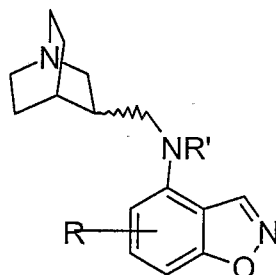
(IVq)
