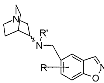
(IIIr)
