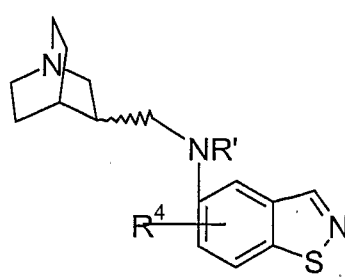
(IVm)
