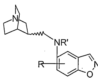
(IVr)
