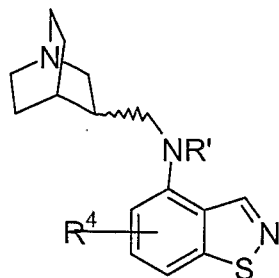
(IVk)
