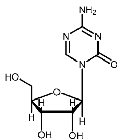
5-Azacytidine.
