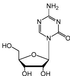
5-Azacytidine.
