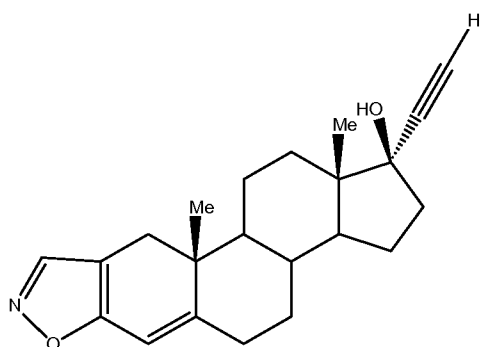
Danazol
