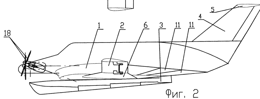
Вид А
