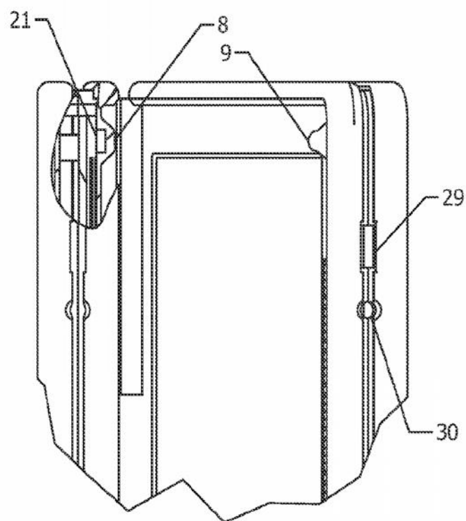
DETAIL 8A SCALE 1 : 1
