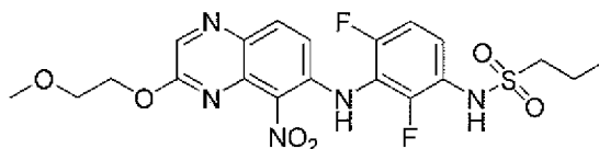
N1-(2,4-difluoro-3-((3-(2-methoxyethoxy)-5-nitro-6-quinoxaliny)amino)phenyl)-1-propanesulfonamide
