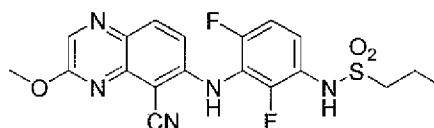
N1-(3-((5-cyano-3-methoxy-6-quinoxaliny)amino)-2,4-difluorophenyl)-1-propanesulfonamide
