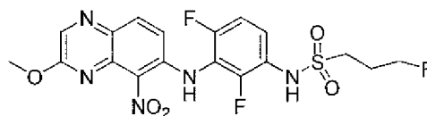
N1-(2,4-difluoro-3-((3-methoxy-5-nitro-6-quinoxaliny)amino)phenyl)-3-fluoro-1-propanesulfonamide
