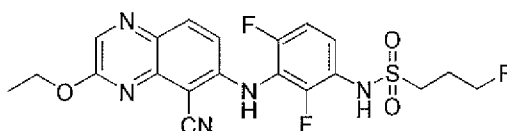
N -(3-(5-cyano-3-ethoxyquinoxalin-6-ylamino)-2,4-difluorophenyl)-3-fluoropropane-1-sulfonamide
