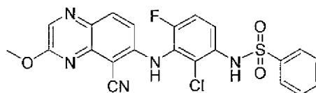
N -(2-chloro-3-(5-cyano-3-methoxyquinoxalin-6-ylamino)-4-fluorophenyl)benzenesulfonamide
