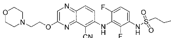
N1-(3-[[5-cyano-3-(2-morpholinoethoxy)-6-quinoxaliny]amino]-2,4-difluorophenyl)-1-propanesulfonamide
