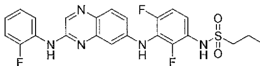
N1-(2,4-difluoro-3-[[3-(2-fluoroanilino)-6-quinoxaliny]amino]phenyl)-1-propanesulfonamide
