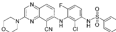
N -(2-chloro-3-(5-cyano-3-morpholinoquinoxalin-6-ylamino)-4-fluorophenyl)benzenesulfonamide
