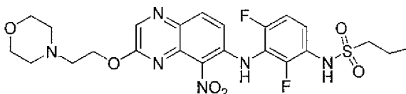
N1-(2,4-difluoro-3-((3-(2-morpholinoethoxy)-5-nitro-6-quinoxaliny)amino)phenyl)-1-propanesulfonamide
