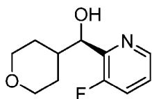
Enantiomer a1
