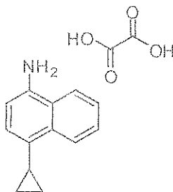
(Compound 8-A).
