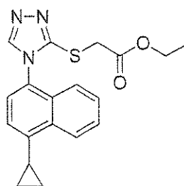
(Compound 2-A).
