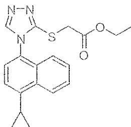
(Compound 2-A).
