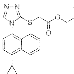
(Compound 2-A).
