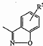
(b-10)
