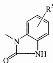
(b-11)
