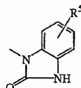
(b-11)
