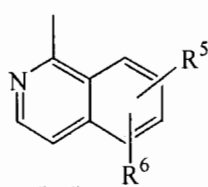
(b-6)
