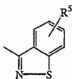
(b-9)
