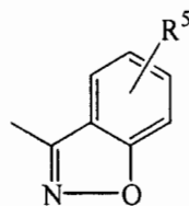
(b-10)
