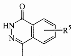
(b-5)
