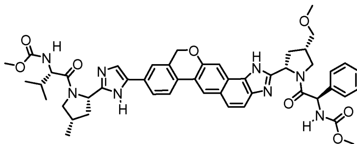
methyl ((2S)-1-((2S,4S)-2-(5-(2-((2S,4S)-1-((2R)-2-((methoxycarbonyl)amino)-2-phenylacetyl)-4-(methoxymethyl)pyrrolidin-2-yl)-1,11-dihydroisochromeno[4',3':6,7]naphtho[1,2-d]imidazol-9-yl)-1H-imidazol-2-yl)-4-methylpyrrolidin-1-yl)-3-methyl-1-oxobutan-2-yl)carbamate
