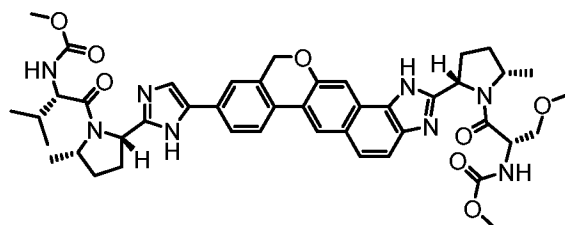
methyl [(2S)-1-{(2S,5S)-2-[5-(2-{(2S,5S)-1-[N-(methoxycarbonyl)-O-methyl-L-seryl]-5-methylpyrrolidin-2-yl)-1,11-dihydroisochromeno[4',3':6,7]naphtho[1,2-d]imidazol-9-yl)-1H-imidazol-2-yl]-5-methylpyrrolidin-1-yl}-3-methyl-1-oxobutan-2-yl]carbamate
