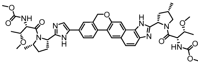
methyl [(2S,3R)-3-methoxy-1-[(2S,5S)-2-[9-(2-{(2S,5S)-1-[N-(methoxycarbonyl)-O-methyl-L-threonyl]-5-methylpyrrolidin-2-yl]-1H-imidazol-5-yl)-1,11-dihydroisochromeno[4',3':6,7]naphtho[1,2-d]imidazol-2-yl]-4-methylpyrrolidin-1-yl]-1-oxobutan-2-yl]carbamate
