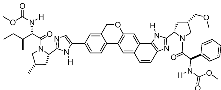
methyl ((1R)-2-[(2S,4S)-2-(9-{2-[(2S,4S)-1-((2S,3R)-2-[(methoxycarbonyl)amino]-3-methylpentanoyl]-4-methylpyrrolidin-2-yl)-1H-imidazol-5-yl)-1,11-dihydroisochromeno[4',3':6,7]naphtho[1,2-d]imidazol-2-yl)-4-(methoxymethyl)pyrrolidin-1-yl]-2-oxo-1-phenylethyl)carbamate
