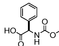
(R)-2-(methoxycarbonylamino)-2-phenylacetic acid
