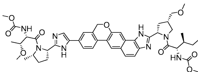
methyl{(2S,3S)-1-[(2S,4S)-2-(9-{2-[(2S,5S)-1-{(2S,3R)-3-methoxy-2-[(methoxy carbonyl)amino]butanoyl}-5-methylpyrrolidin-2-yl]-1H-imidazol-5-yl}-1,11-dihydroisochromeno[4',3':6,7]naphtho[1,2-d]imidazol-2-yl)-4-(methoxymethyl)pyrrolidin-1-yl]-3-methyl-1-oxopentan-2-yl}carbamate
