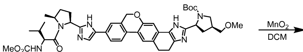
tert-butyl (2S,4S)-2-[9-(2-((2S,5S)-1-[N-(methoxycarbonyl)-L-valyl]-5-methylpyrrolidin-2-yl)-1H-imidazol-5-yl)-1,4,5,11-tetrahydroisochromeno[4',3':6,7]naphtho[1,2-d]imidazol-2-yl]-4-(methoxymethyl)pyrrolidine-1-carboxylate
