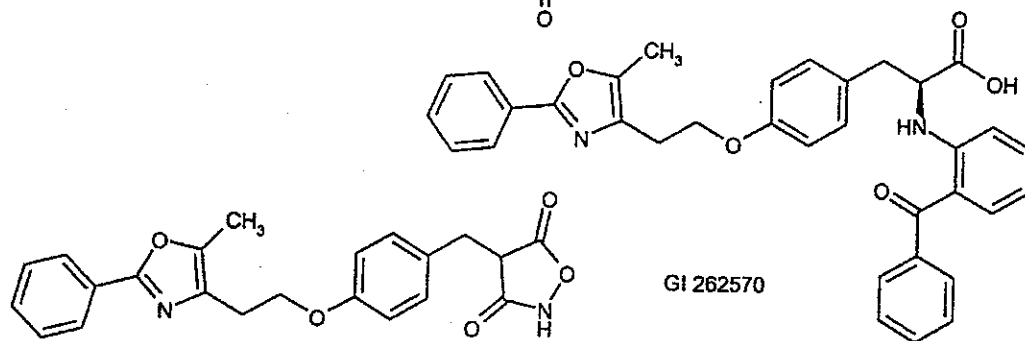
JTT-501
