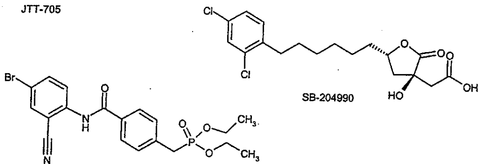
NO-1886
