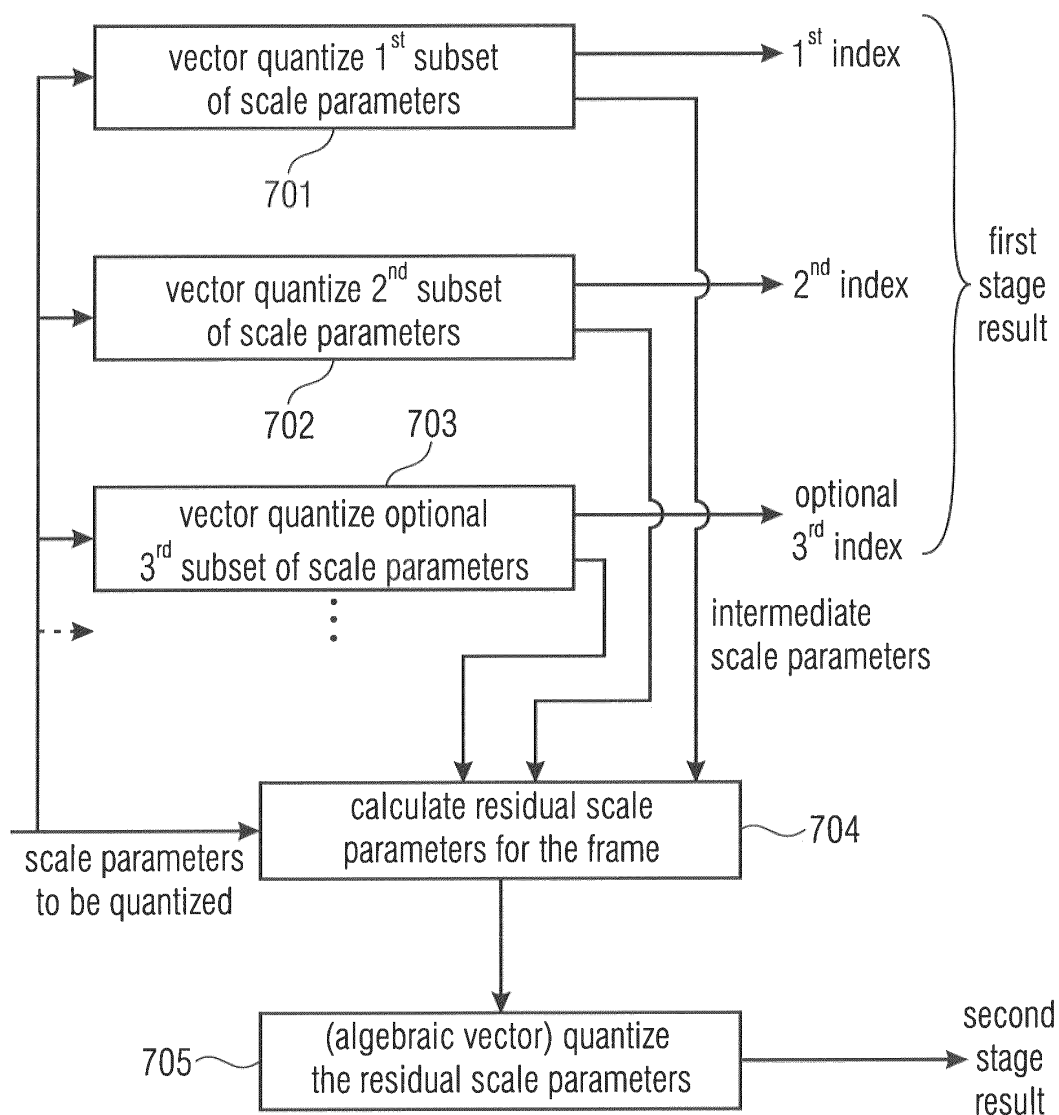
Fig. 7a (FOR SEPARATE SCALE PARAMETERS L, R OR JOINT SCALE PARAMETERS M)
