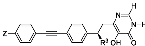
Formula (IVa).
