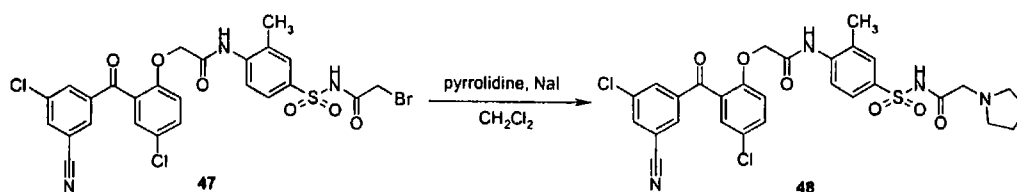
Scheme VI
