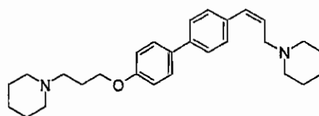
(Z)-1-(3-{[4'-(3-piperidinoprop-1-en-1-yl)biphenyl-4-yl]oxy}propyl)piperidine
