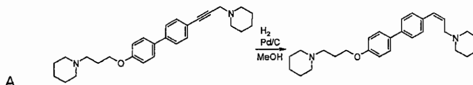
(Z)-1-(3-{[4'-(3-piperidinoprop-1-en-1-yl)biphenyl-4-yl]oxy}propyl)piperidine
