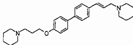
(E)-1-(3-([4'-(3-piperidinoprop-1-en-1-yl)biphenyl-4-yl]oxy)propyl)piperidine
