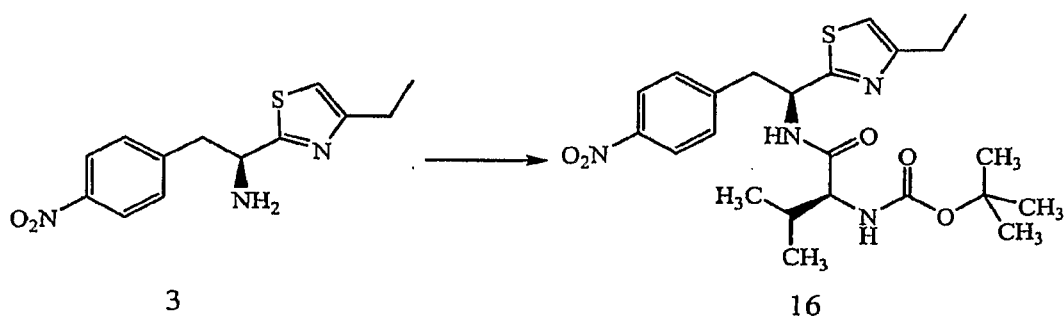
Scheme VI
