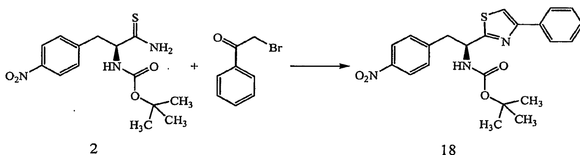
Scheme VI
