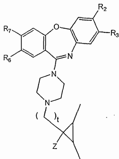
(IVd);
