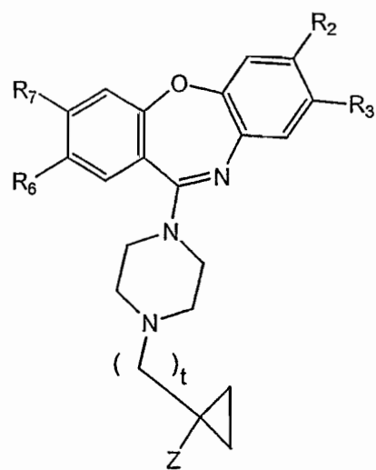
(IVb);
