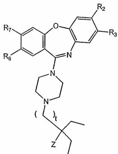
(IVc);
