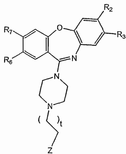
(IVe).
