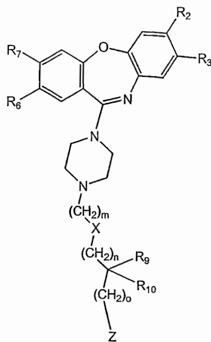
(II)
