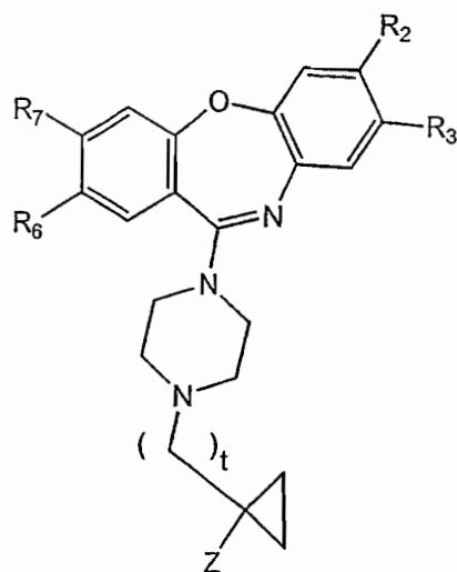
(IVb);
